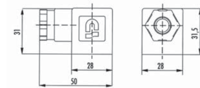
ST 30 Ex ia
